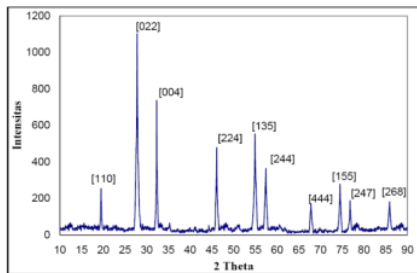
Gambar 4. Difraktogram aurivillius \text{Sr}_2\text{Bi}_3\text{Ti}_4\text{O}_{15} sintesis suhu 200 °C selama 72 jam (Mikrianto et al. , 2016).
