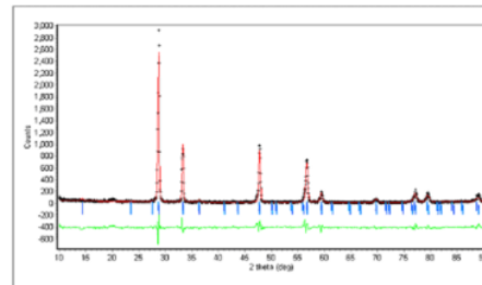
Gambar 3. Pola refinemen struktur aurivillius \text{SrBi}_3\text{Ti}_3\text{O}_{12} (Mikrianto et al. , 2016)
