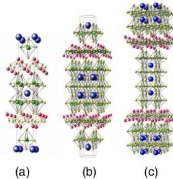
Gambar 1. Struktur Aurivillius berdasarkan jumlah lapis oktahedral pada lapisan perovskit (a). 2 lapis (b). 3 lapis (b). 4 lapis (Mikrianto et al. , 2016)
