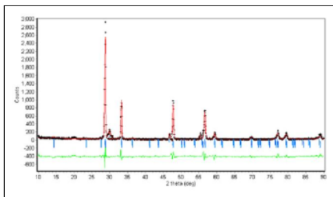
Gambar 9. Pola refinemen struktur aurivillius \text{Sr}_3\text{Bi}_3\text{Ti}_6\text{O}_{21} (Mikrianto et al. , 2016).
