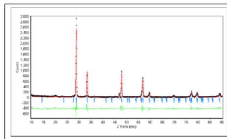
Gambar 7. Pola refinemen struktur aurivillius \text{Sr}_3\text{Bi}_3\text{Ti}_5\text{O}_{18} (Mikrianto et al. , 2016).
