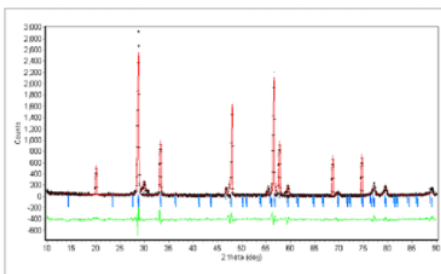
Gambar 5. Pola refinemen struktur aurivillius \text{Sr}_2\text{Bi}_3\text{Ti}_4\text{O}_{15} (Mikrianto et al. , 2016).
