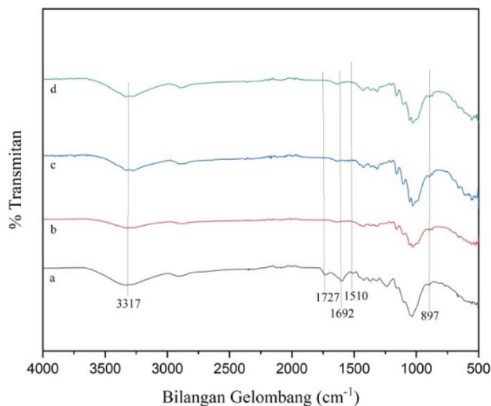
Gambar 2. Spektre FTIR a) pelepah sagu; b) hasil delignifikasi 5%; c) hasil delignifikasi 7,5%; d) hasil delignifikasi 10%
