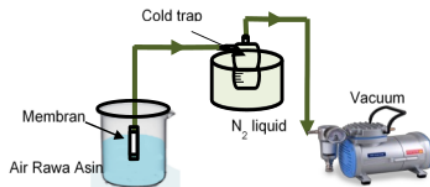
Gambar 2. Rangkaian Alat Pervaporasi
