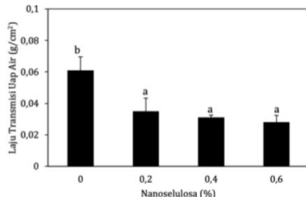
Gambar 6. Data laju transmisi uap air bioplastik
