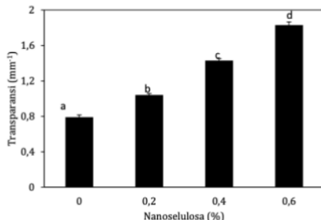
Gambar 5. Data transparansi bioplastik
