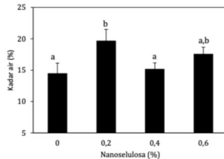
Gambar 3. Data kadar air bioplastik
