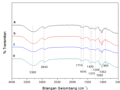
Gambar 2. Spektra FTIR bioplastik dengan penambahan a) 0%; b) 0,2%; c) 0,4%; dan d) 0,6% nanoselulosa
