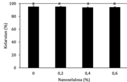
Gambar 7. Data kelaurutan bioplastik
