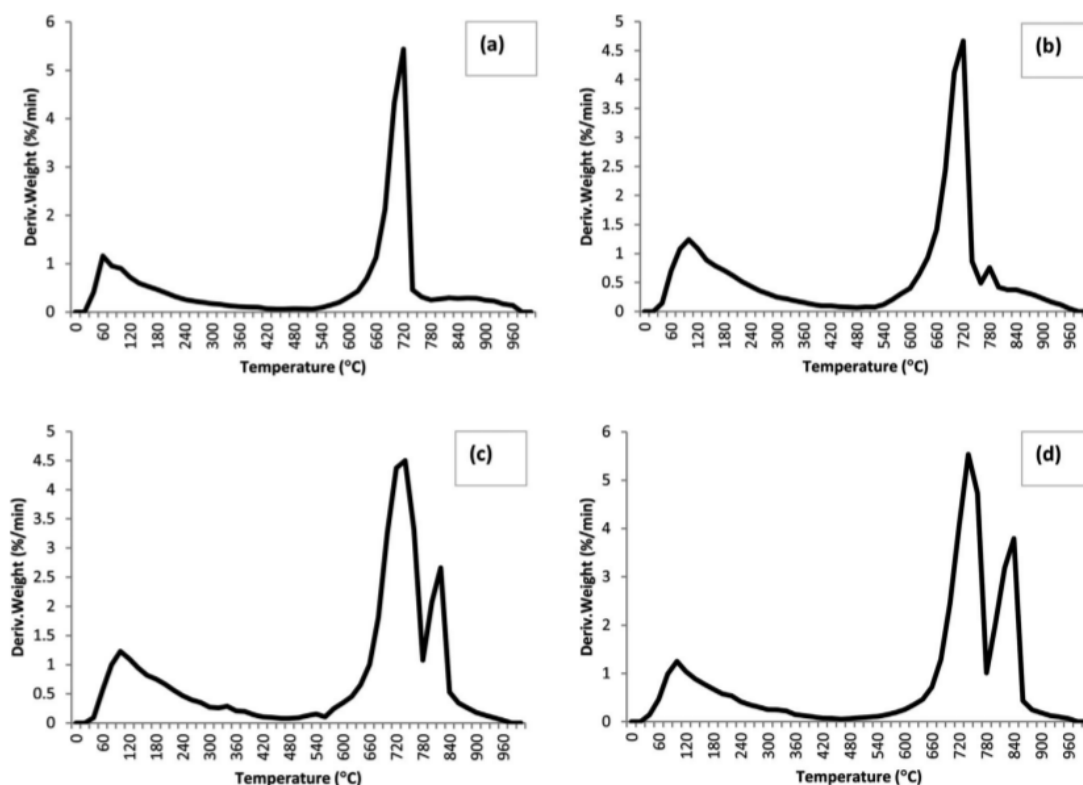
Figure 6. DTG curves of prepared catalysts: (a) SZ, (b) 1Ni-SZ, (c) 3Ni-SZ, (d) 5Ni-SZ.
