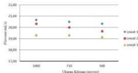
Gambar 6. Grafik Hubungan antara Flowrate (mL/s) terhadap Variasi Ukuran Kitosan (micron)
