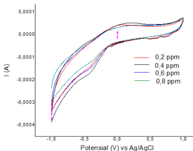
Gambar 5. Voltametri siklik dengan variasi larutan glukosa
