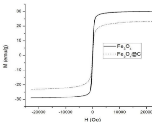
Gambar 2. Kurva histeresis nanopartikel \text{Fe}_3\text{O}_4 dan nanokomposit \text{Fe}_3\text{O}_4@\text{C}
