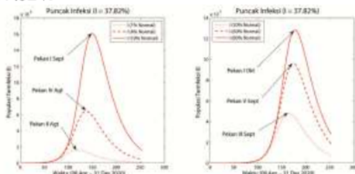
Gambar 3. Perkiraan puncak kasus Infeksi ( I ) = 37.82%
