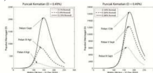
Gambar 4. Perkiraan puncak kasus Kematian ( D ) = 0.49%
