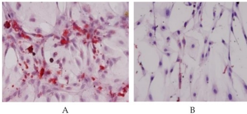
Gambar 10. Sel preadiposit yang mengalami maturasi. (A. tanpa inhibitor STAT3, B. dengan inhibitor STAT3)
