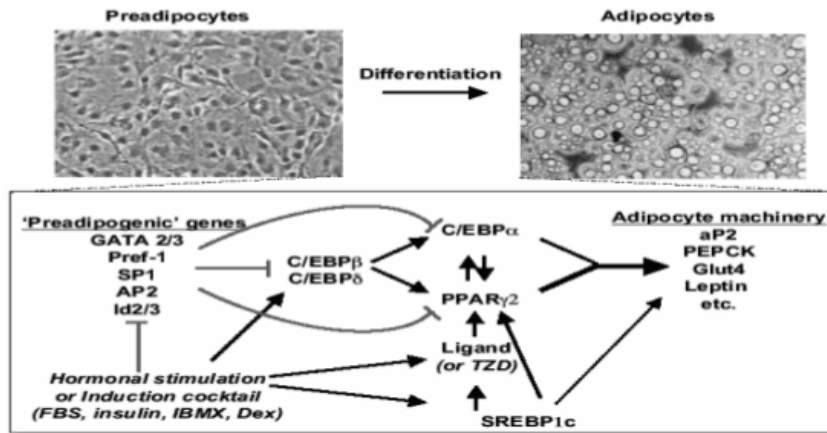
Gambar 5. Pengaruh stimulasi hormonal dalam proses diferensiasi sel adiposit (Sumber: Sethi & Puig 2007)
