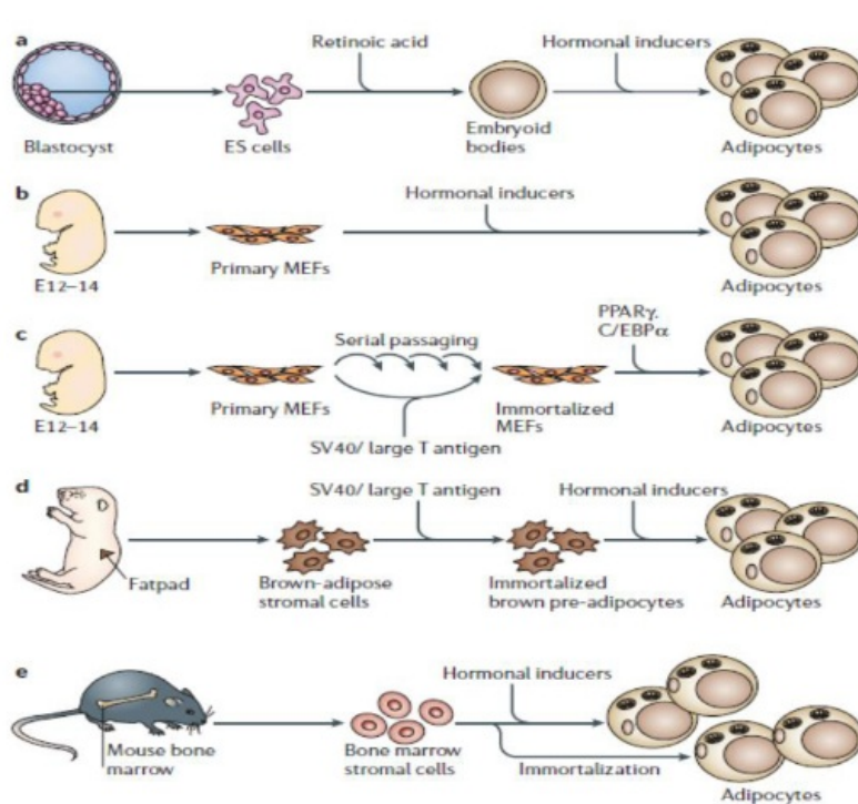
Gambar 3. Beberapa model seluler yang dapat digunakan untuk mempelajari adipogenesis yang melibatkan hampir seluruh tahap perkembangan (Sumber: Rosen & MacDougald 2006)
