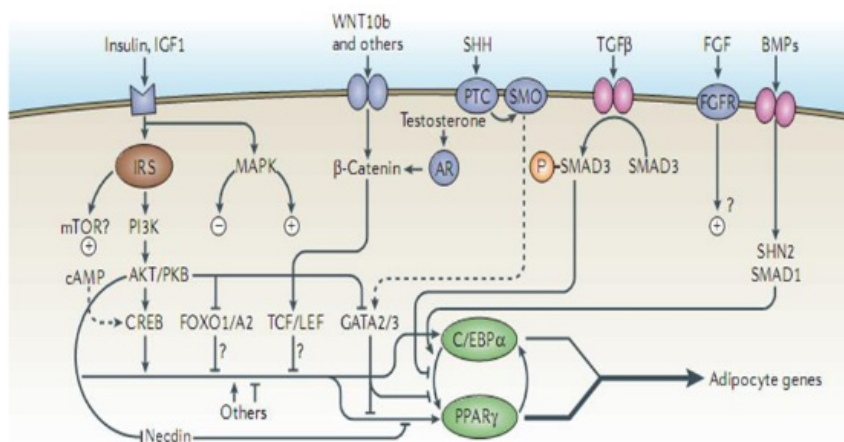
Gambar 6. Regulasi adipogenesis oleh faktor-faktor ekstraseluler (Sumber: Rosen & MacDougla 2006)
